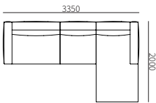
B28ZH-4 3350*2000*655mm 131.9*78.7*25.8"
