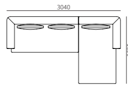
尺寸: 3040*1800*700mm 编码: T33ZH-2
