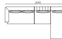
尺寸: 3640*1800*700mm 编码: T33ZH-3
